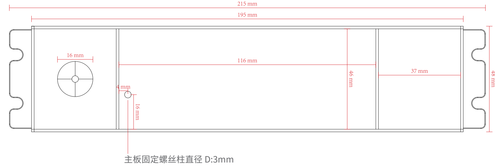
顶视图
