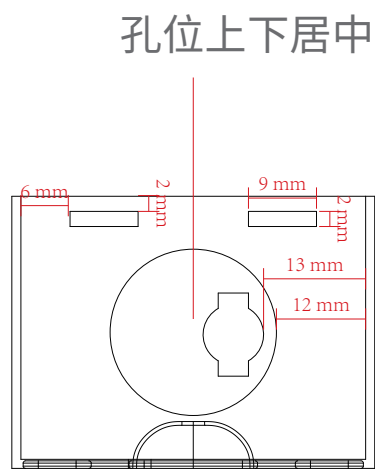
左视图
